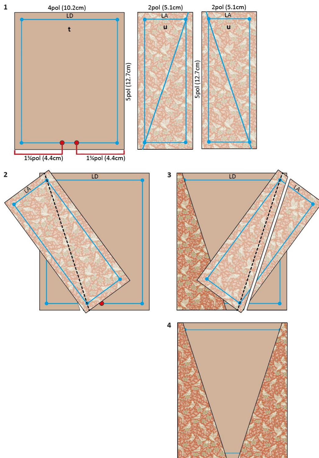
Fig K Fazer a unidade t+u+u para a secção torácica
