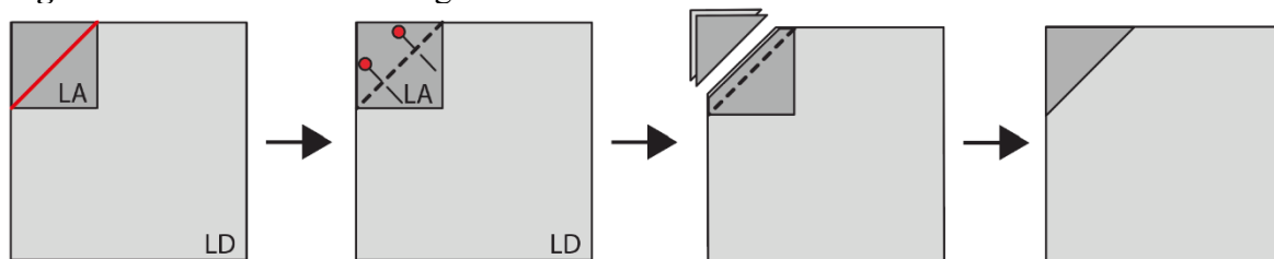
Fig E Fazer uma unidade triangular de canto
