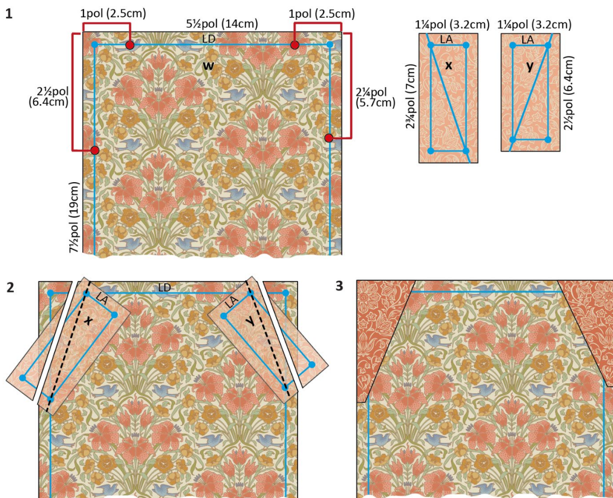
Fig M Fazer unidade w+x+y para secção de saia
