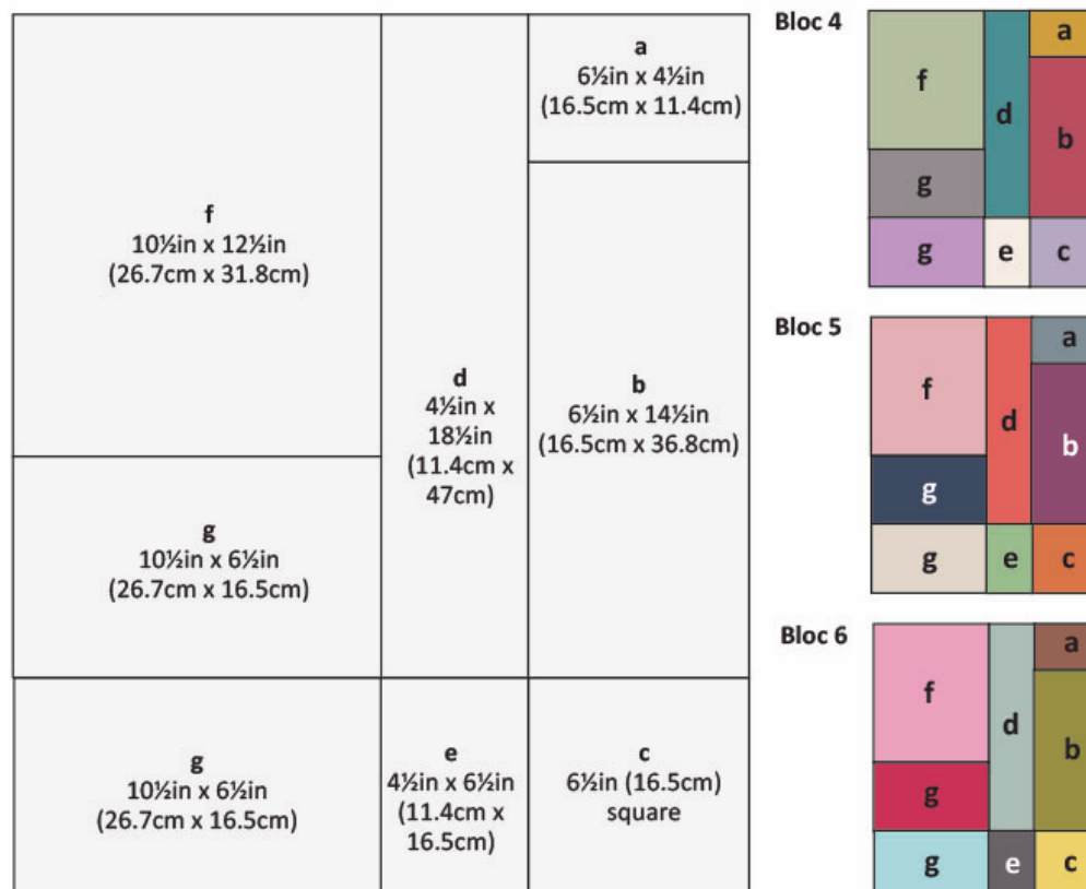
Fig. D Plan et découpe des Blocs 4, 5 et 6 Les dimensions comprennent les marges de couture.
