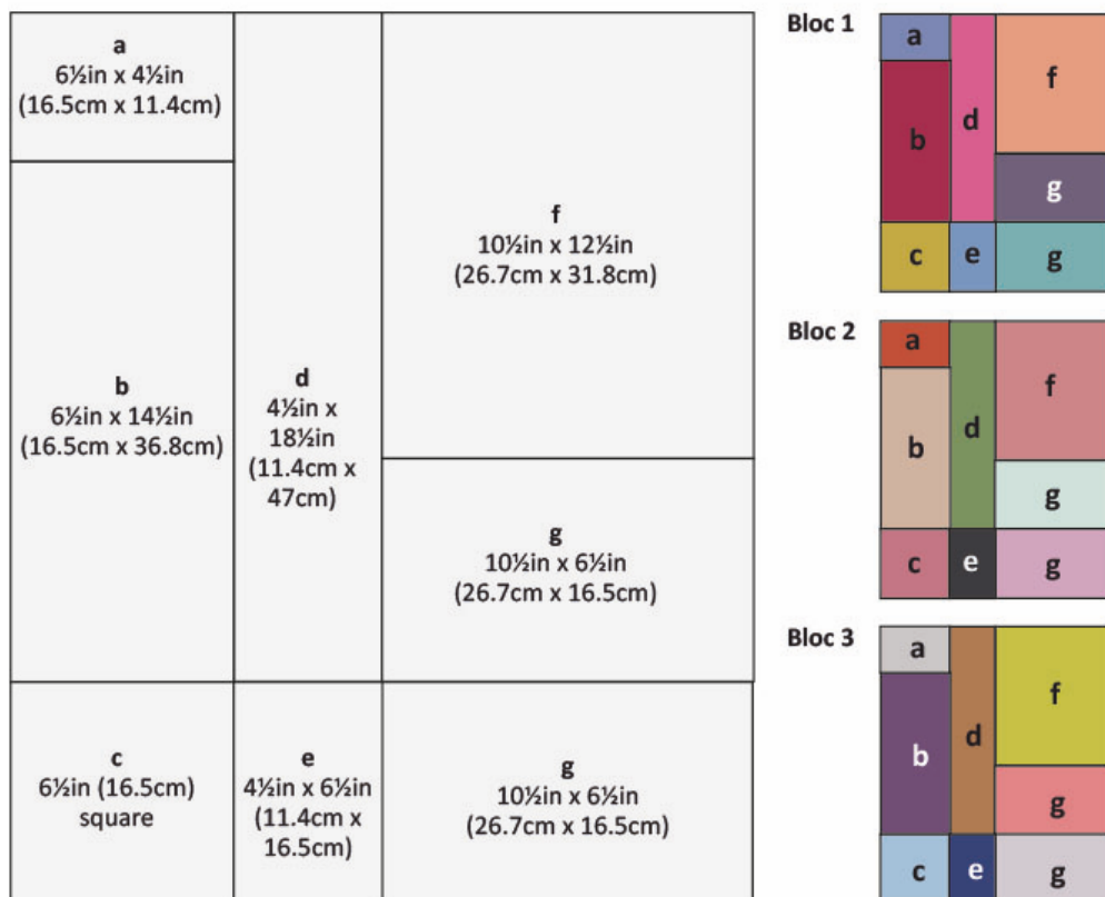
Fig. C Plan et découpe des Blocs 1, 2 et 3 Les dimensions comprennent les marges de couture.
